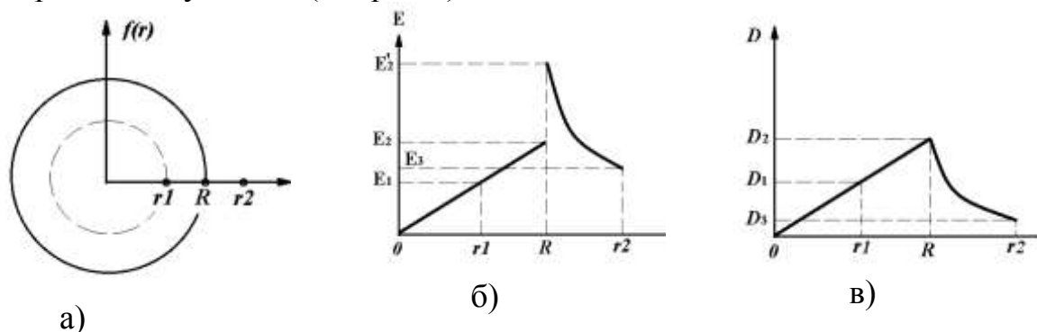
Рисунок 2- Диэлектрический шар радиусом R с зарядом, равномерно распределенным по объему - (а), и графики зависимости от расстояния r напряженности электростатического поля E - (б) и электрического смещения D - (в)
