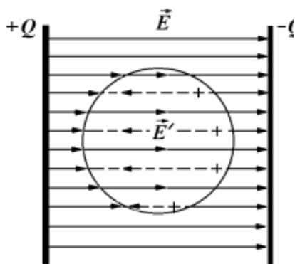
Рисунок 1- Структура электрического поля в диэлектрическом объекте, помещенном в однородное электрическое поле
